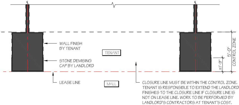
PLAN - TENANT TYPE A2
