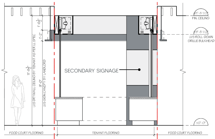
SECTION (N.T.S.)
