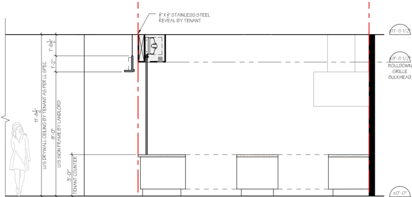
SECTION (N.T.S.)
