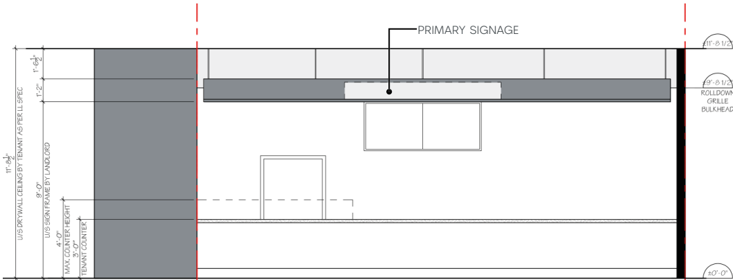
FRONT ELEVATION (N.T.S.)
