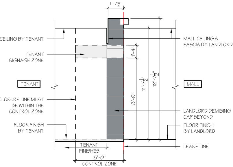
SECTION - TENANT TYPE A2
