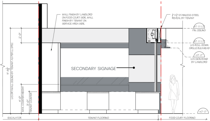
SECTION (N.T.S.)
