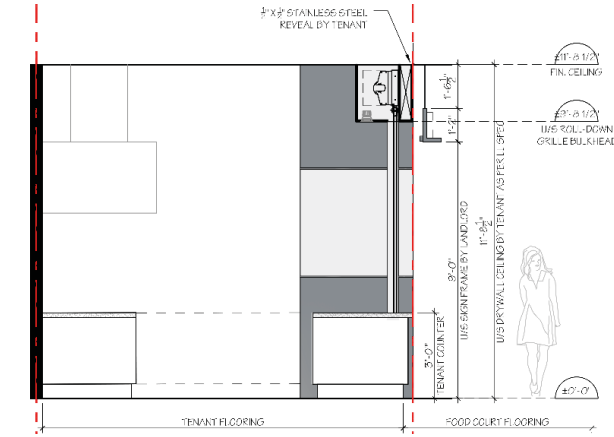
SECTION (N.T.S.)
