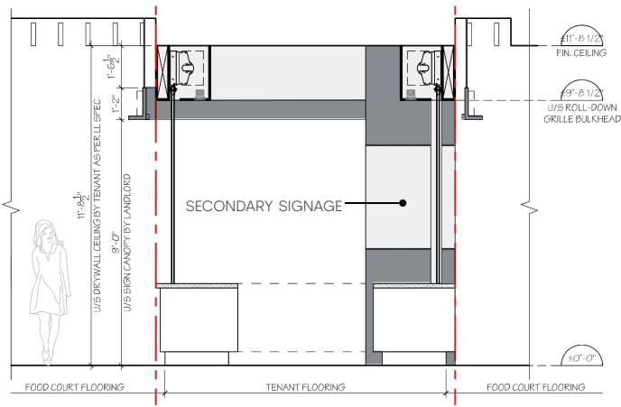
SECTION (N.T.S.)
