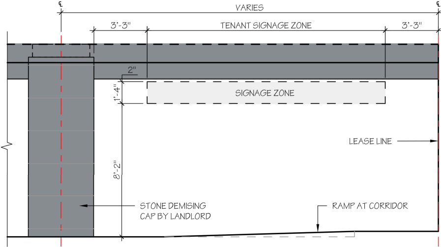
ELEVATION - TENANT TYPE A3
