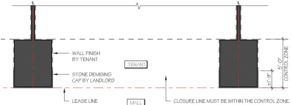
ELEVATION - TENANT TYPE A2
