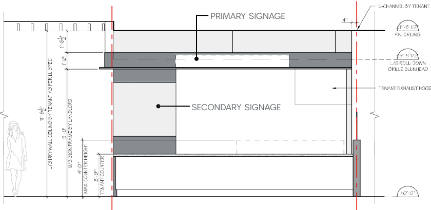
SECTION (N.T.S.)
