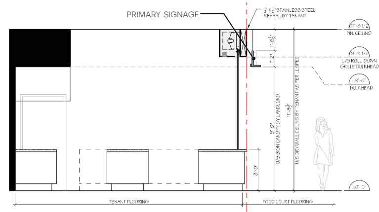
SECTION (N.T.S.)
